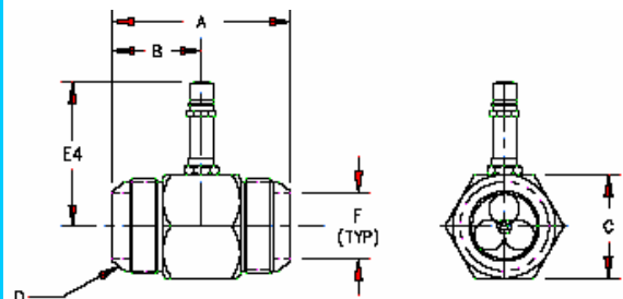
Abmaße größerer Turbinen und oder mit Flanschanschluss auf Anforderung.
